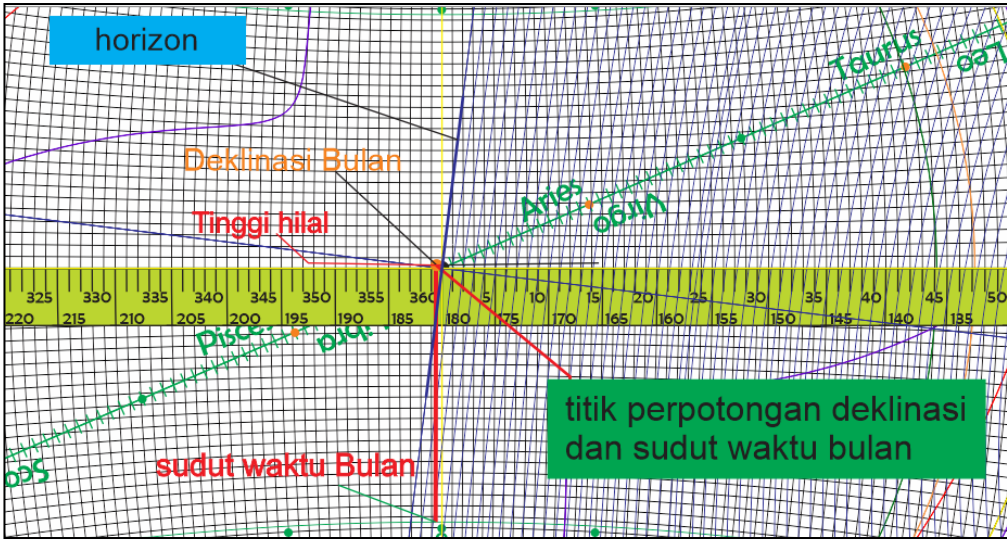
Gambar 4.19. Mencari Ketinggian Hilal dari nilai deklinasi dan sudut waktu Bulan
