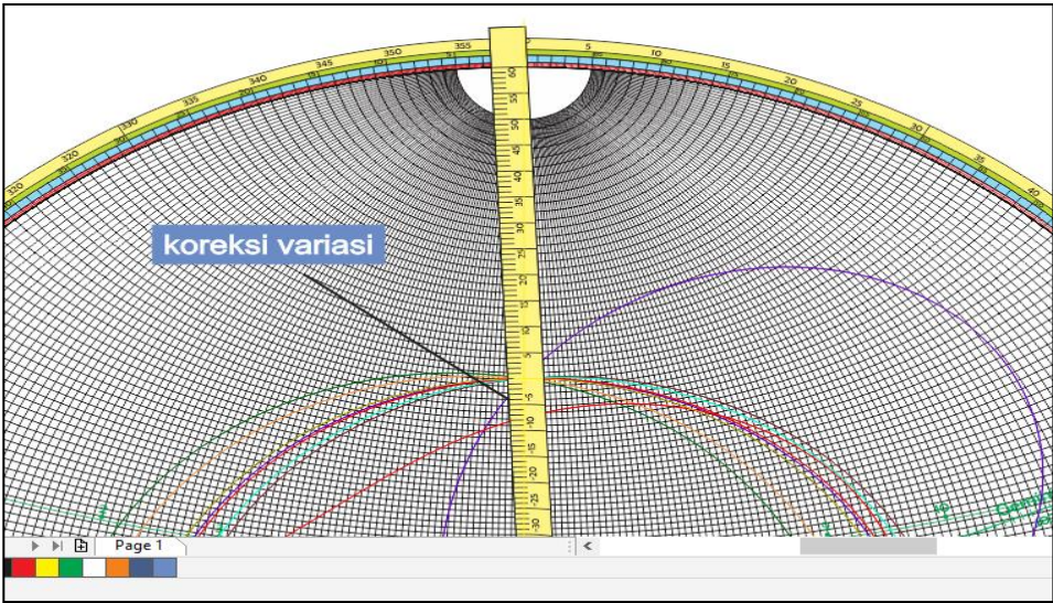
Gambar 4.13. Mencari Koreksi Variasi
