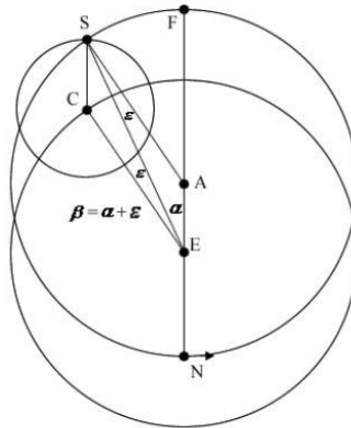
Gambar 2.6 Geometri teori Pergerakan Matahari Ptolomeus. Sudut \epsilon disebut prostaphaeresis dan sudut \alpha merupakan posisi Matahari dilihat dari Bumi.
