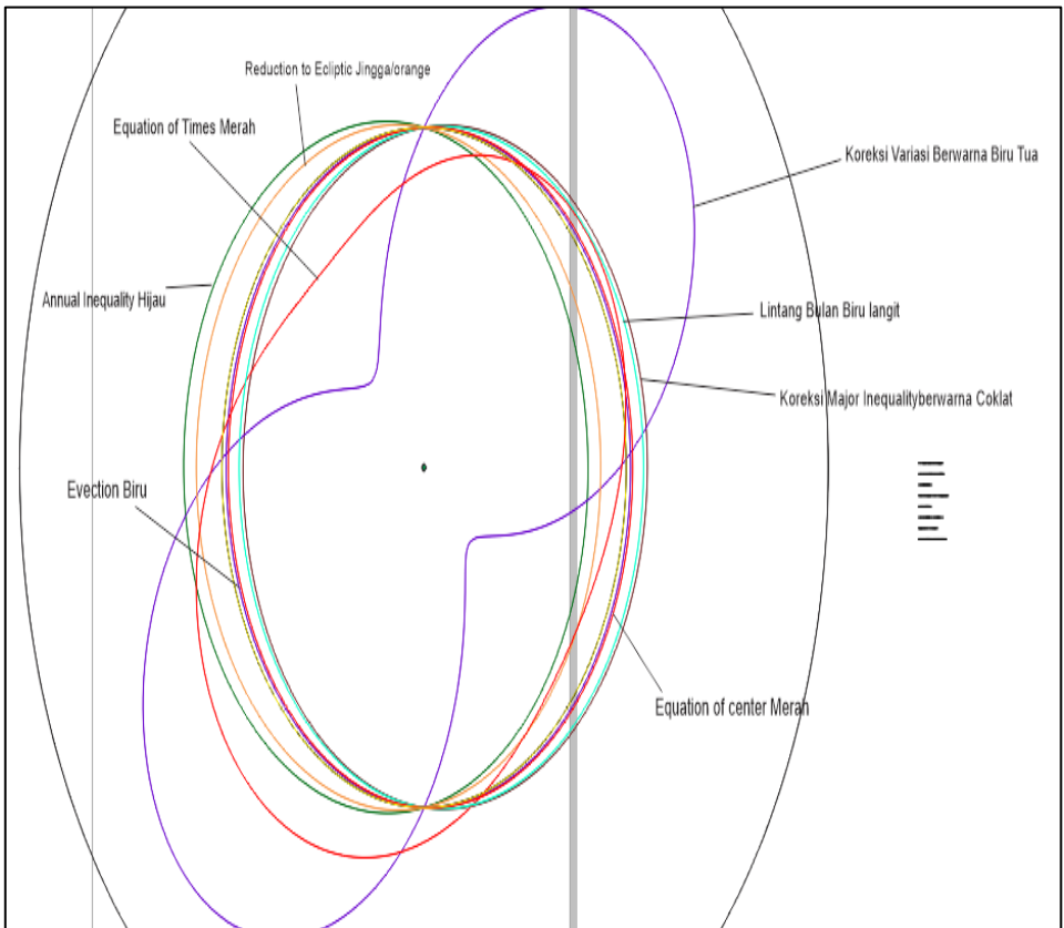
Gambar 4.2. Kurva koreksi Pergerakan Bulan, Matahari, dan Equation of time
