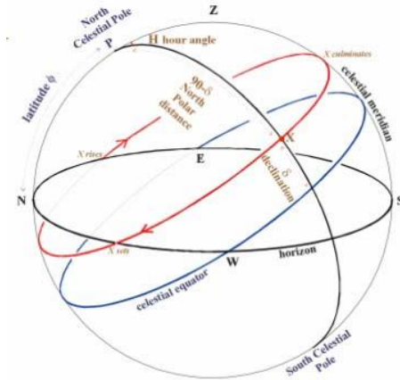
Gambar 2.4 Bola langit sistem koordinta ekuator Hour Angle dan Deklinasi
