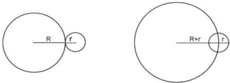
Gambar 2.7. Lingkaran dengan jari-jari ( R ) adalah lingkaran deferent dan lingkaran jari-jari ( r ) adalah lingkaran epicycle .
