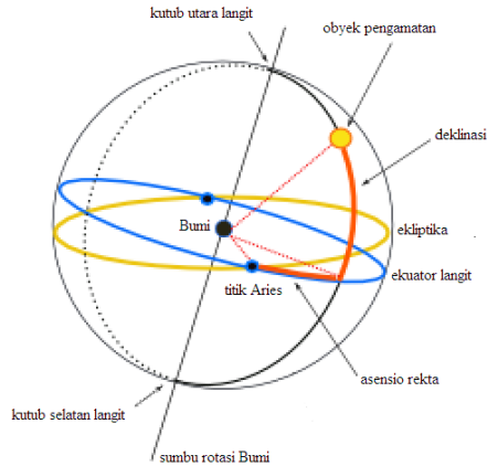
Gambar 2.3. Bola langit sistem equator Aksensio rekta dan Deklinasi
