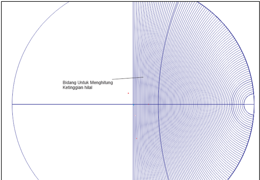
Gambar 4.6. Bidang Plot dan Transformasi Koordinat
