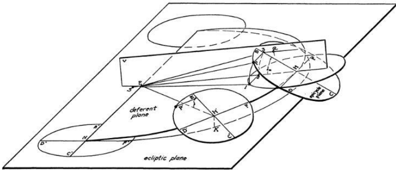
Gambar 3.3. Lingkaran lintang Bulan
