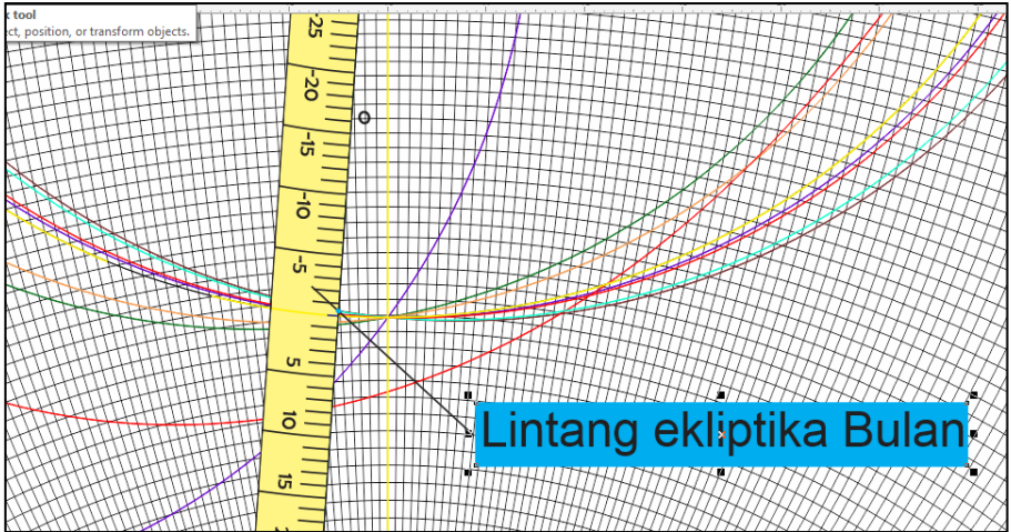
Gambar 4.16. Mencari Lintang Bulan
