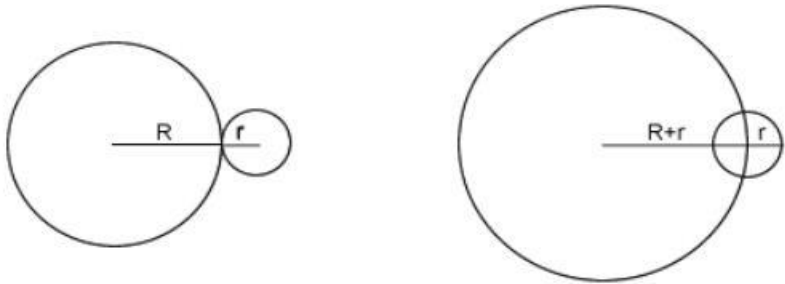
Gambar 3.2. Lingkaran dengan jari-jari ( R ) adalah lingkaran deferent dan lingkaran jari-jari ( r ) adalah lingkaran epicycle.
