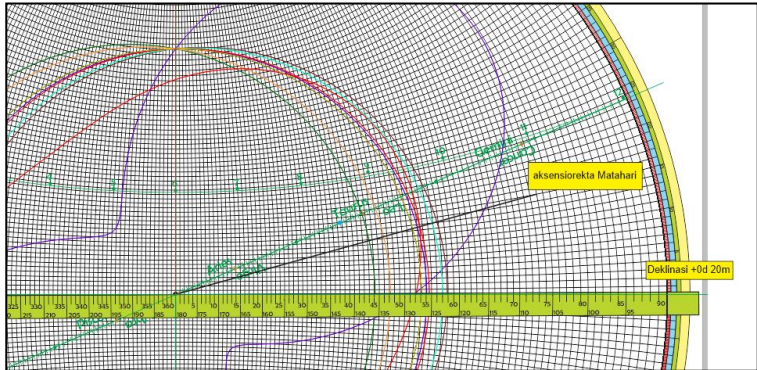
Gambar 4.10. Mencari Deklinasi dan Aksensiorekta Matahari
