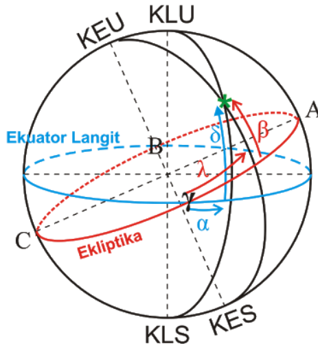
Gambar 2.2. Bola langit sistem koordinat ekliptika
