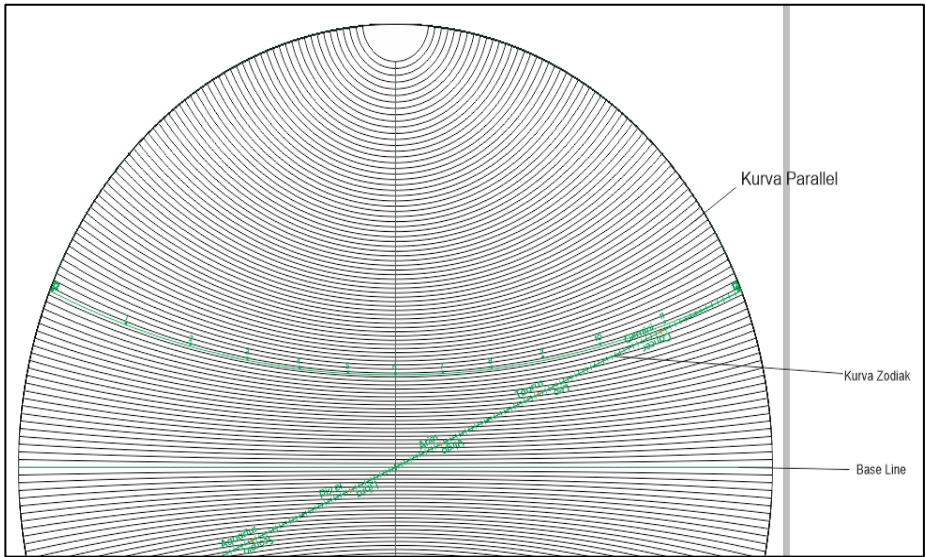
Gambar 4.3. Kurva Paralel, Ekliptika, dan Ekuator 25
