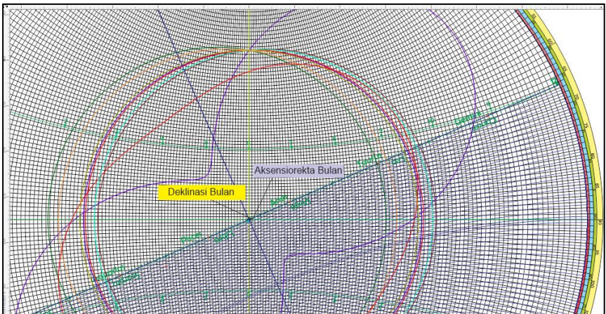
Gambar 4.17. peletakan titik pada lintang ekliptika bulan negatif dan bujur ekliptika Bulan sekitar 178^\circ 52' .
