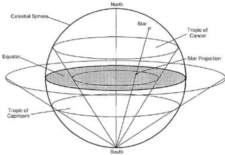
Gambar 2.9. Prinsip proyeksi stereografik
