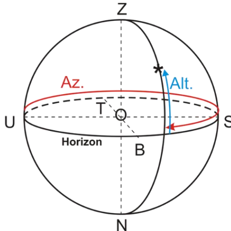
Gambar 2.5 Bola langit sistem koordinat Horizon
