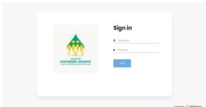
Gambar 1. Menu Login
