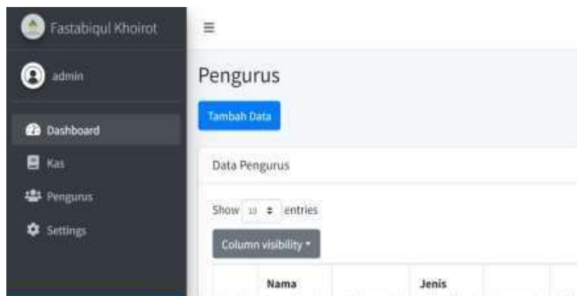
Gambar 2. Menu Pilihan
