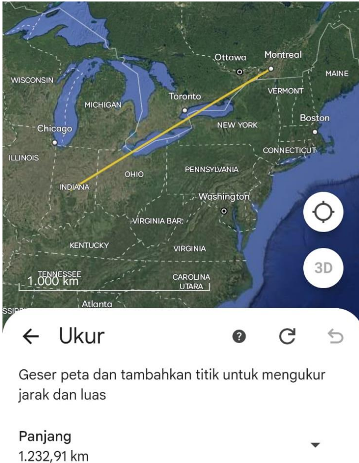
Gambar 4.1: Jarak antara Montreal dengan Indiana pada Google Earth
