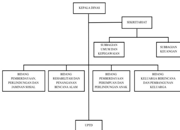
Gambar 2. Struktur DINSOSP3AKB
