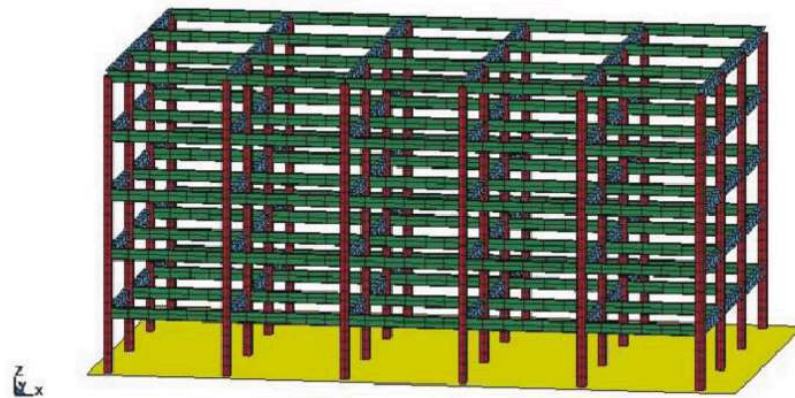
Gambar 4.7. Rigid frame
